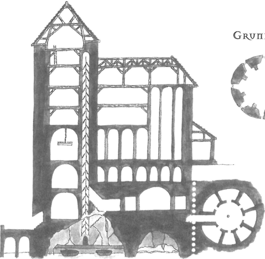
SEITENANSICHT DES GROßEN TURMS UND DES PALAS SOWIE GRUNDRISS DES ZELLENTRAKTES
