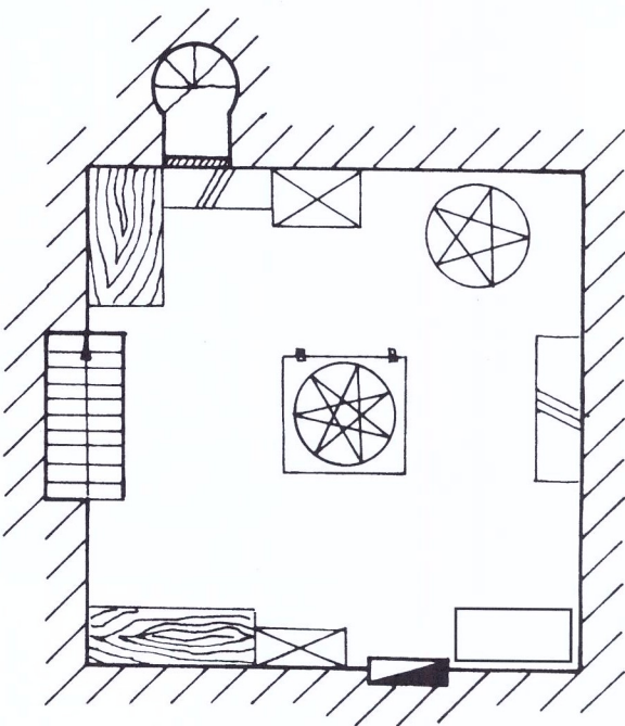
2. Kellergeschoß
