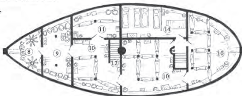
Unterdeck
