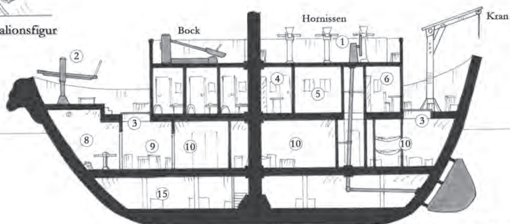
Schnitt
