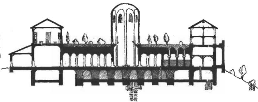
Seitenriß
