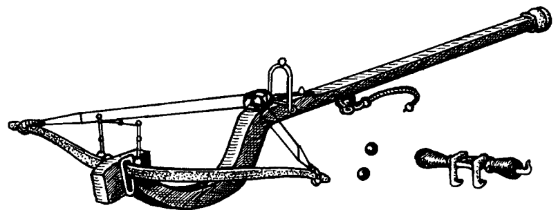
Abb. 82: Balläster oder Schnepper zur Vogeljagd, mit Bleikugeln und Spannknobel; man beachte die Visiereinrichtung; aus dem Besitz des Answin von Rabenmund
